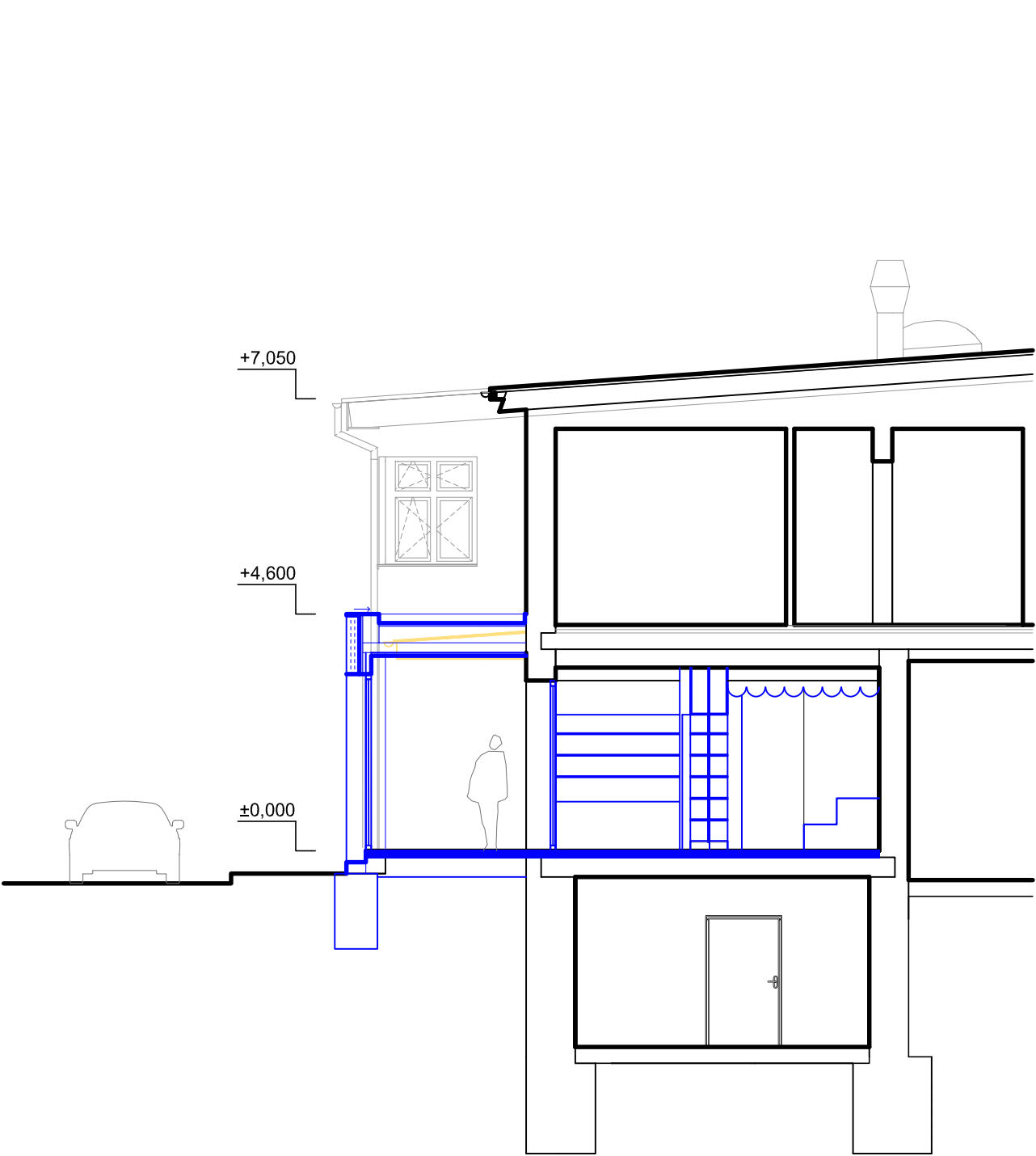
řezopohled vstupu do knihovny
